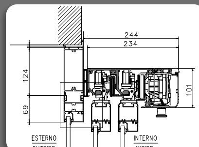
Telescopische versie met montage op dwarsbalk
