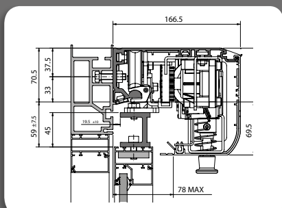
Met zelfdragend profiel en afstandshouders
